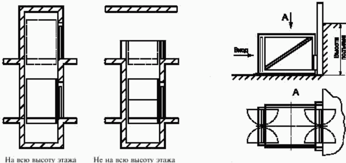
Рисунок 2 — Подъемная платформа без ограждения шахты
