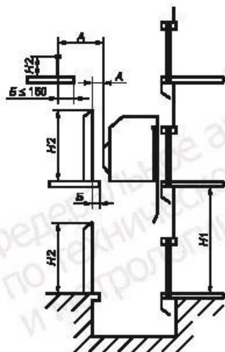
А — расстояние до движущихся элементов лифта; Б — расстояние между ограждением и краем межэтажных перекрытий, ступеней и площадок; Н1 — высота ограждения со стороны этажной площадки; Н2 — высота ограждения с остальных сторон
