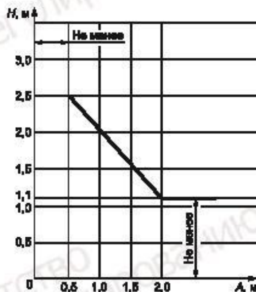
А — расстояние от движущихся элементов лифта; Н — высота ограждения
