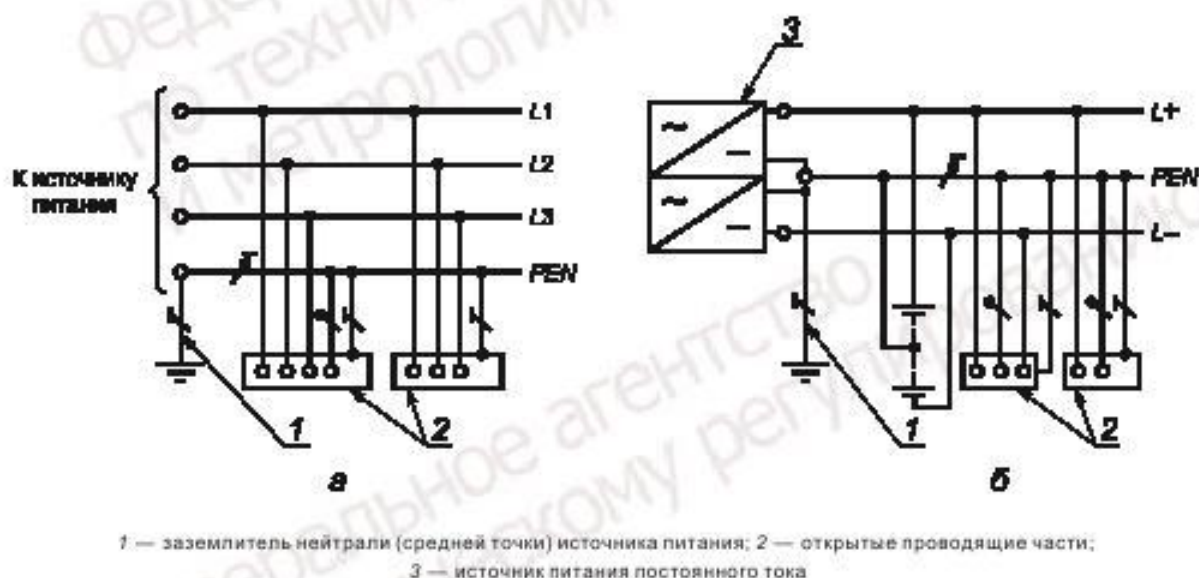
Рисунок 6 — Система TN-C переменного(а) и постоянного(б) тока. Нулевой защитный и нулевой рабочий проводники совмещены в одном проводнике
