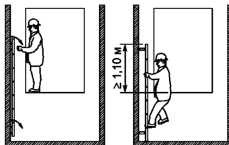
Тип 2а – Выдвижная лестница приямка
