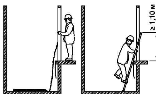
Тип 4 – Складная лестница приямка
