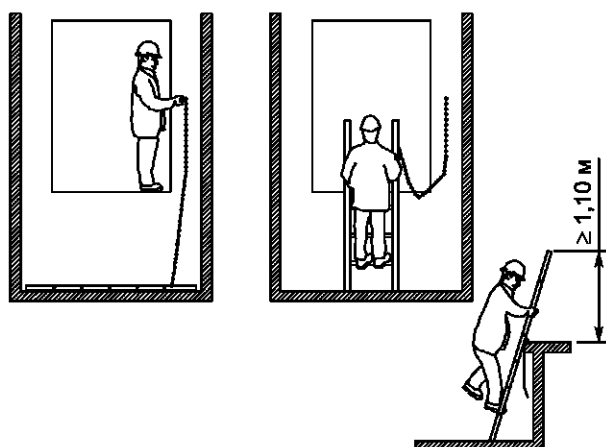
Тип 3б – Передвижная лестница приямка
