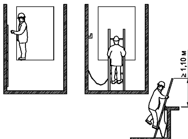
Тип 3а – Передвижная лестница приямка
