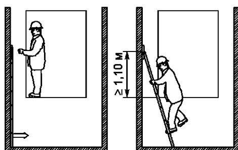
Тип 2б – Выдвижная лестница приямка
