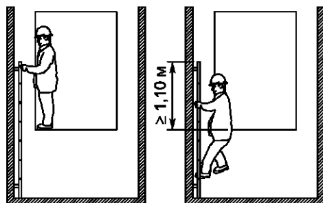
Тип 1 – Фиксированная лестница приямка
